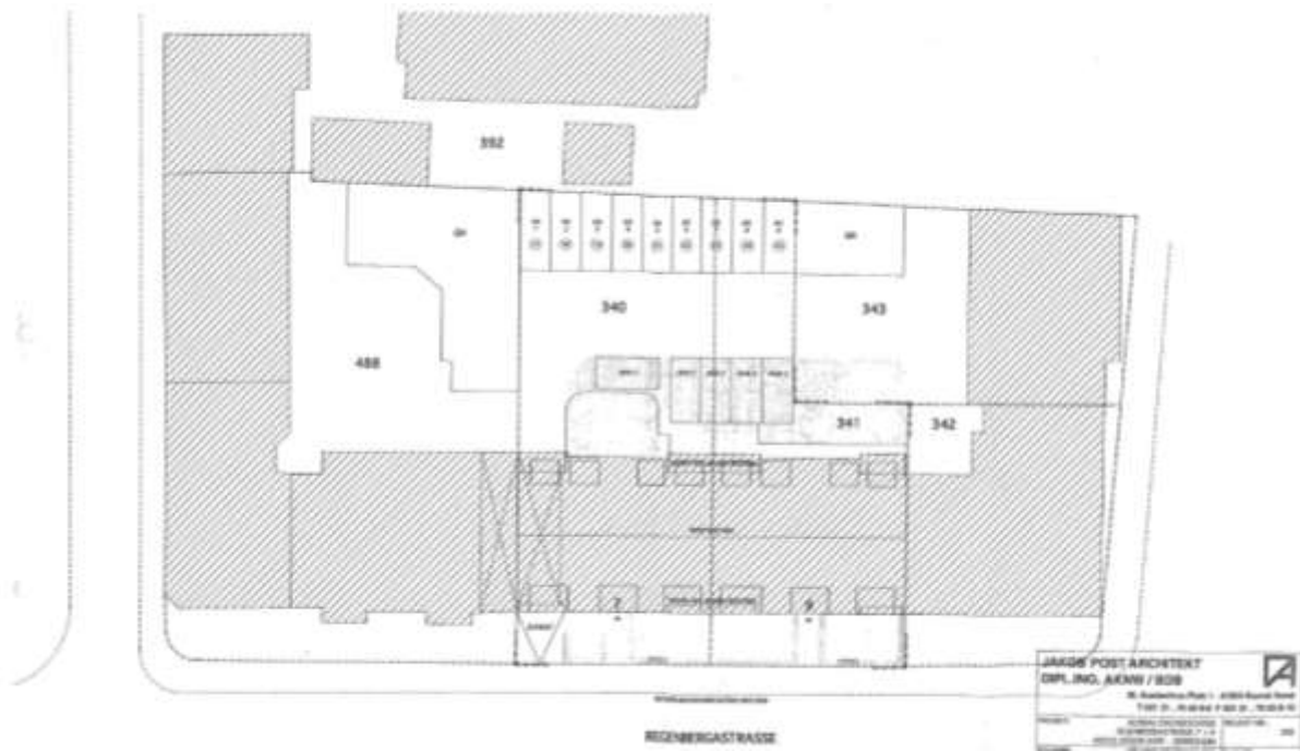
Lageplan
