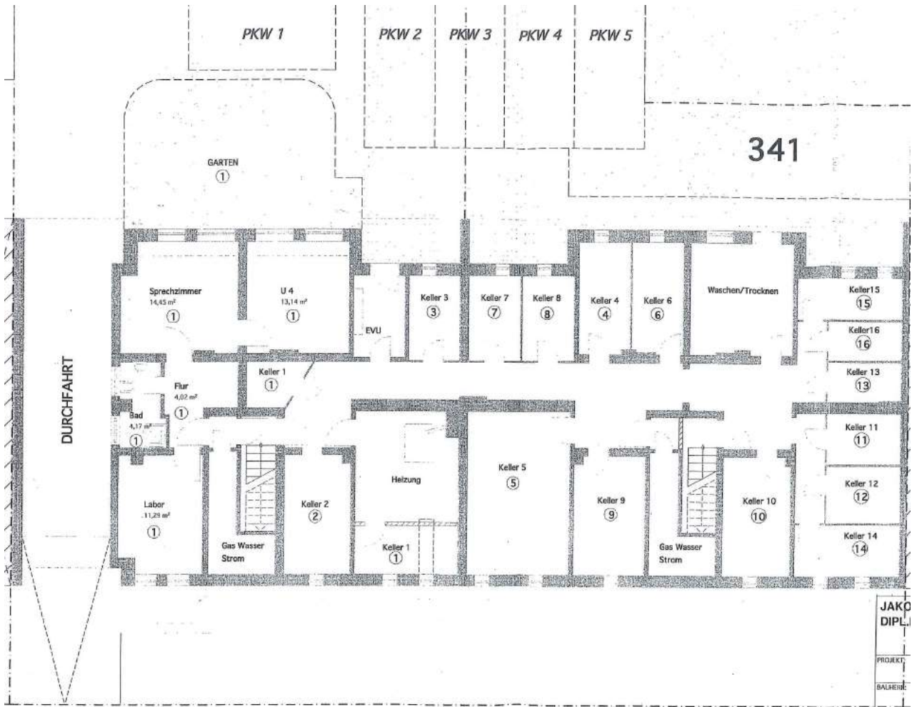
Grundriss Keller 13, Stellplatz 3
