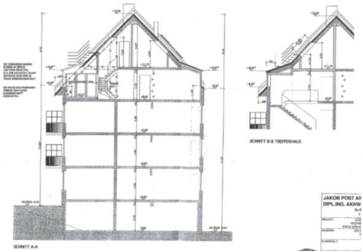
Schnitt
