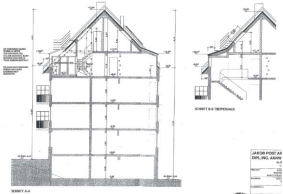
Schnitt
