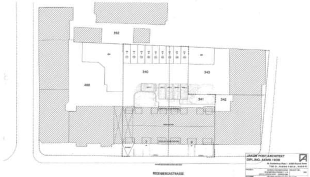
Lageplan
